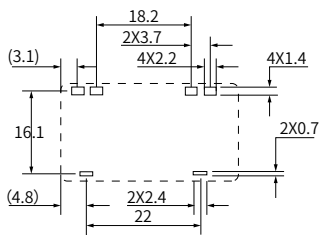
安装孔尺寸 PCB Layout (底视 Bottom View)
