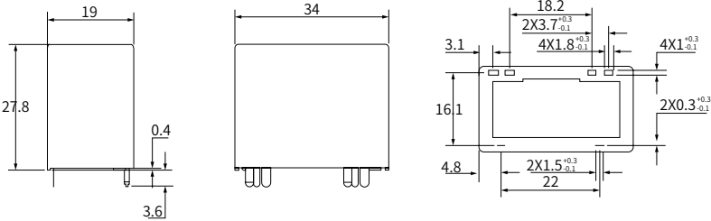
外形尺寸 Profile Dimension
