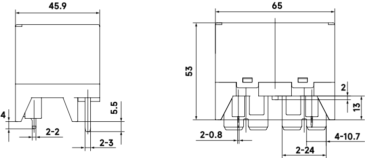
外形尺寸 Profile Dimension
