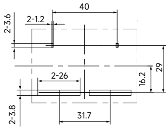
安装孔尺寸 PCB Layout (底视 Bottom View)
