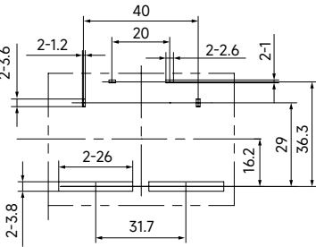
安装孔尺寸 PCB Layout (底视 Bottom View)
