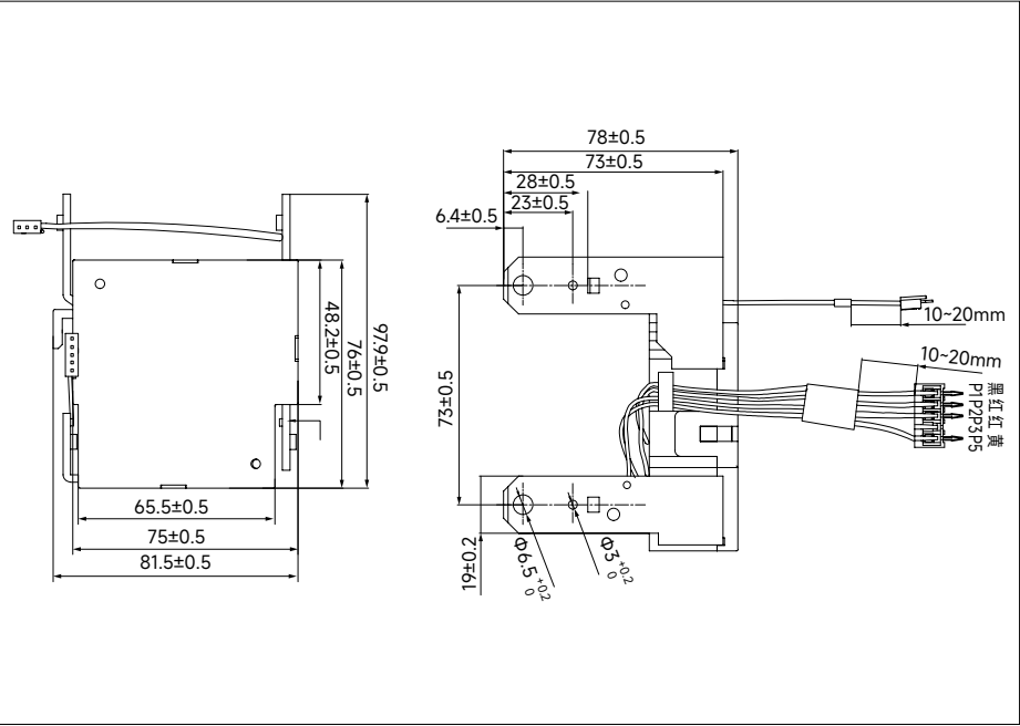
外形尺寸 PROFILE DIMENSION
