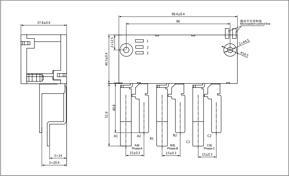
外形尺寸 PROFILE DIMENSION
