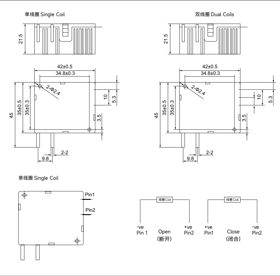
外形尺寸 PROFILE DIMENSION
