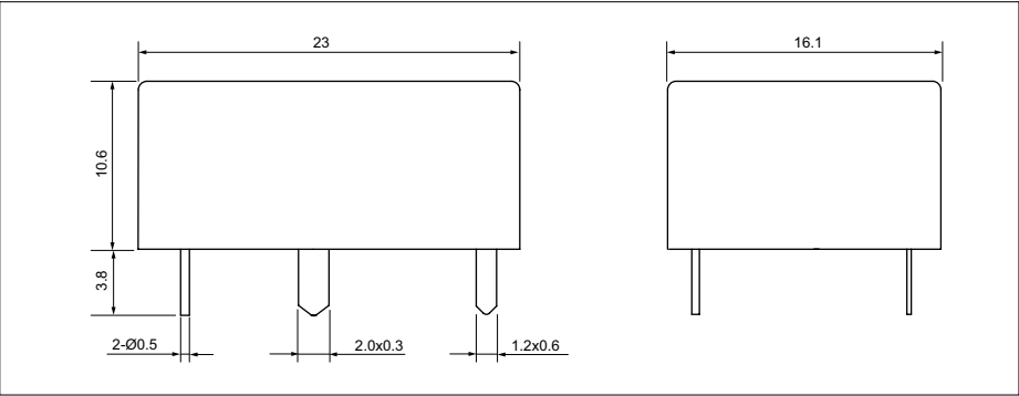
外形尺寸 PROFILE DIMENSION
