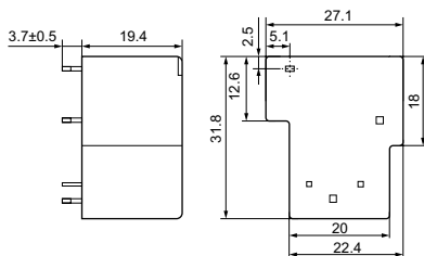
外形尺寸 Profile Dimension
