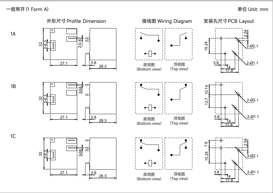
外形尺寸，接线图，安装孔尺寸 PROFILE DIMENSION, WIRING DIAGRAM AND PCB LAYOUT
